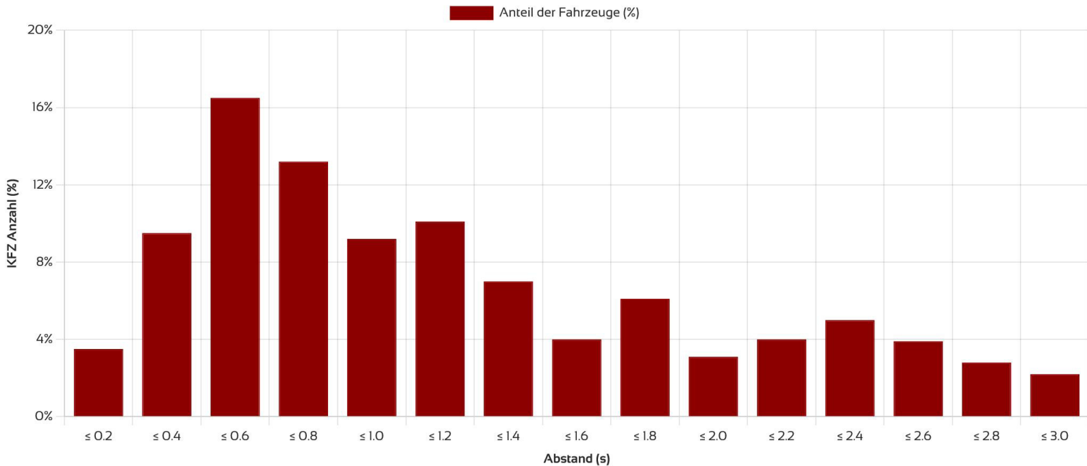
KFZ Anzahl (%) vs. Abstand (s)
