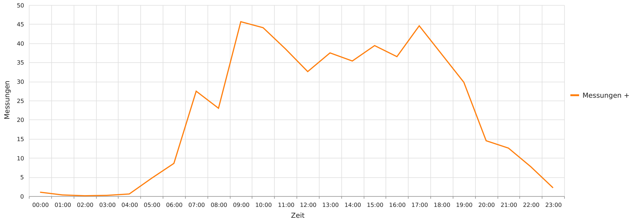
Straße Grand-Couronne-Allee, beide Fahrtrichtungen, 30 km/h Beschränkung Gemittelte Anzahl an Messwerten vs. Uhrzeit
