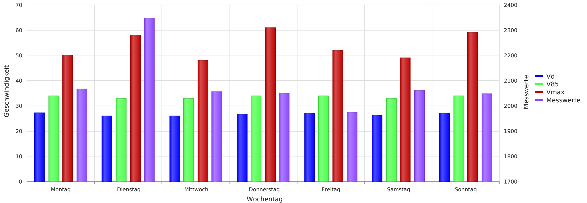
Straße Grand-Couronne-Allee, beide Fahrtrichtungen, 30 km/h Beschränkung Vd, V85, Vmax, Anzahl der Messwerte vs. Wochentag
