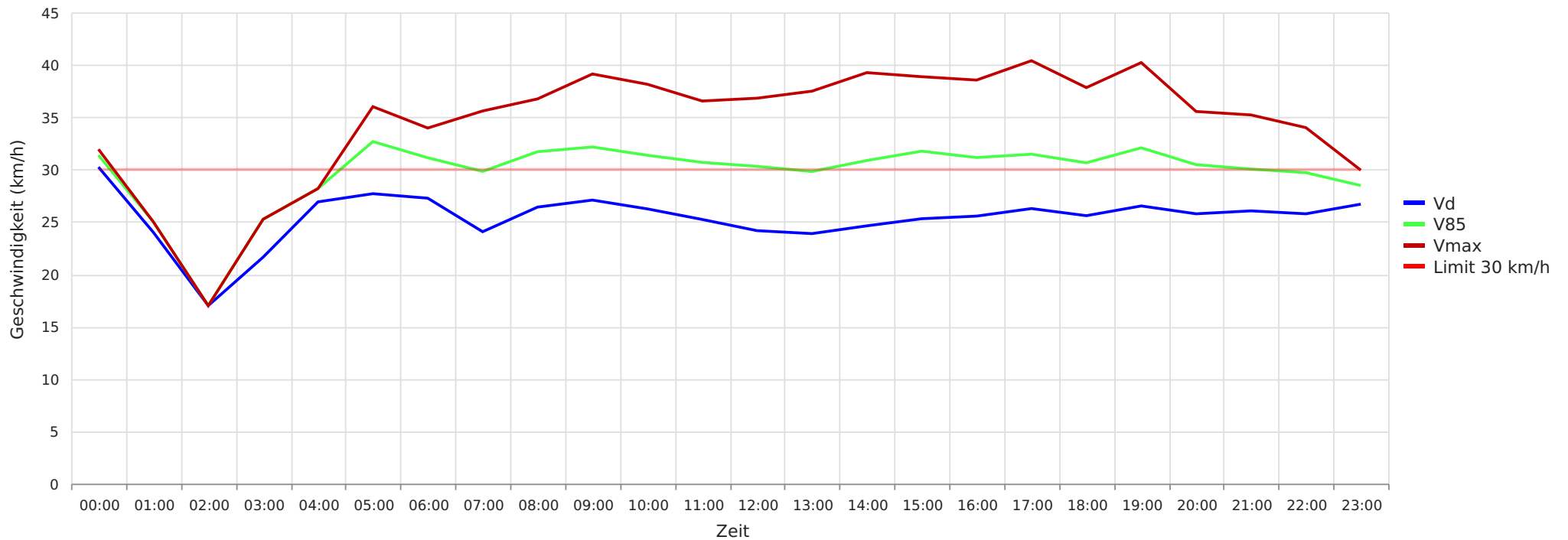
Straße Grand-Couronne-Allee, beide Fahrtrichtungen, 30 km/h Beschränkung Vd, V85, Vmax vs. Uhrzeit
