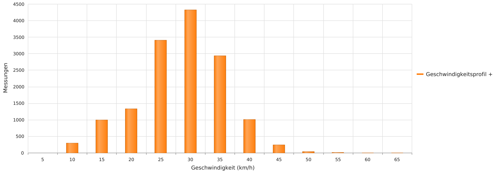
Straße Grand-Couronne-Allee, beide Fahrtrichtungen, 30 km/h Beschränkung Anzahl der Messwerte vs. Geschwindigkeit
