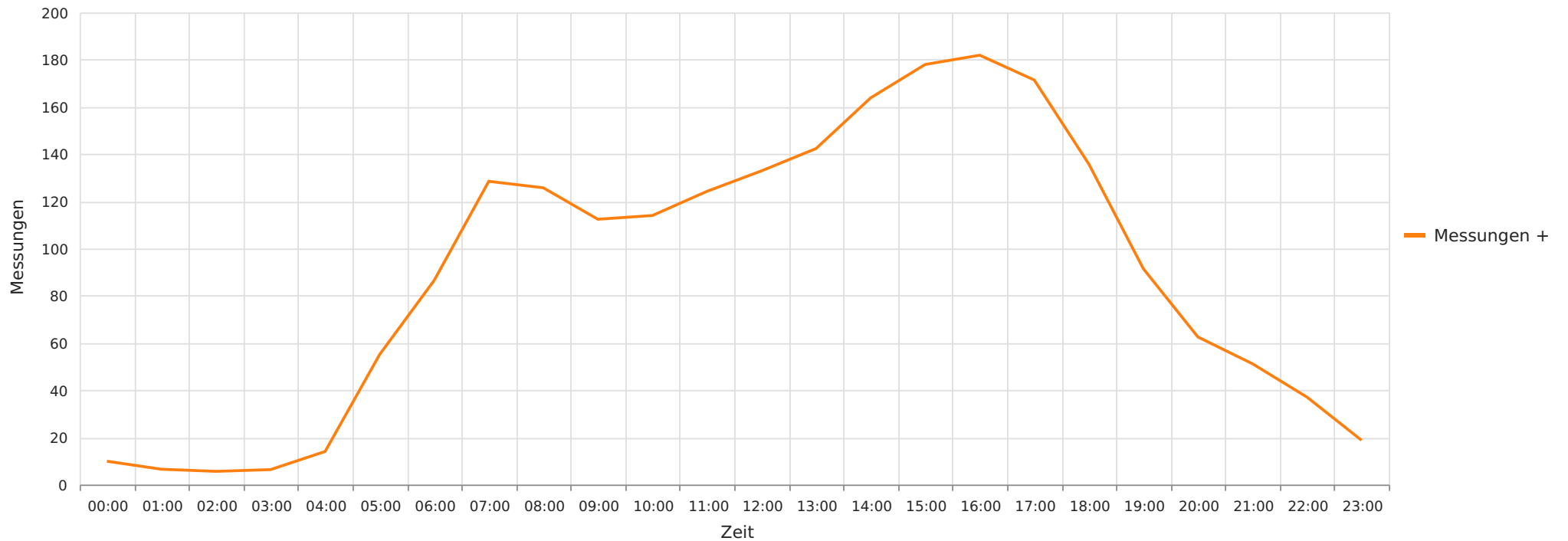
K 251 Lathwehren, beide Fahrtrichtungen, 70 km/h Gemittelte Anzahl an Messwerten vs. Uhrzeit
