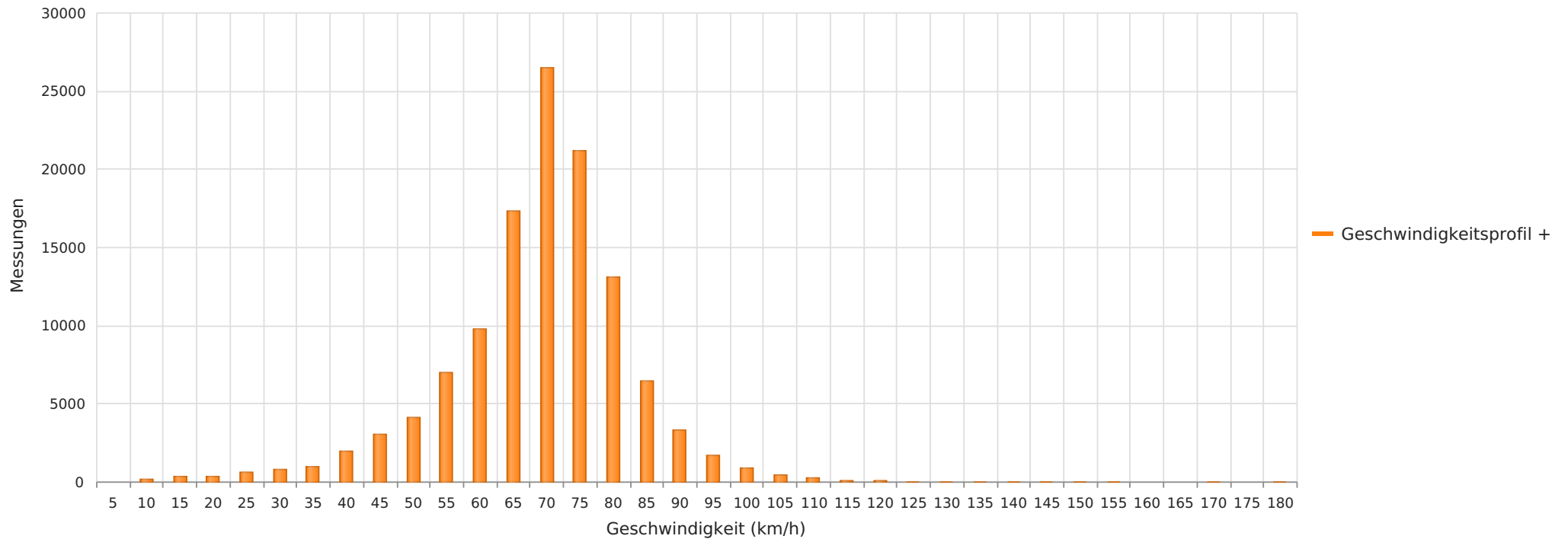
K 251 Lathwehren, beide Fahrtrichtungen, 70 km/h Anzahl der Messwerte vs. Geschwindigkeit
