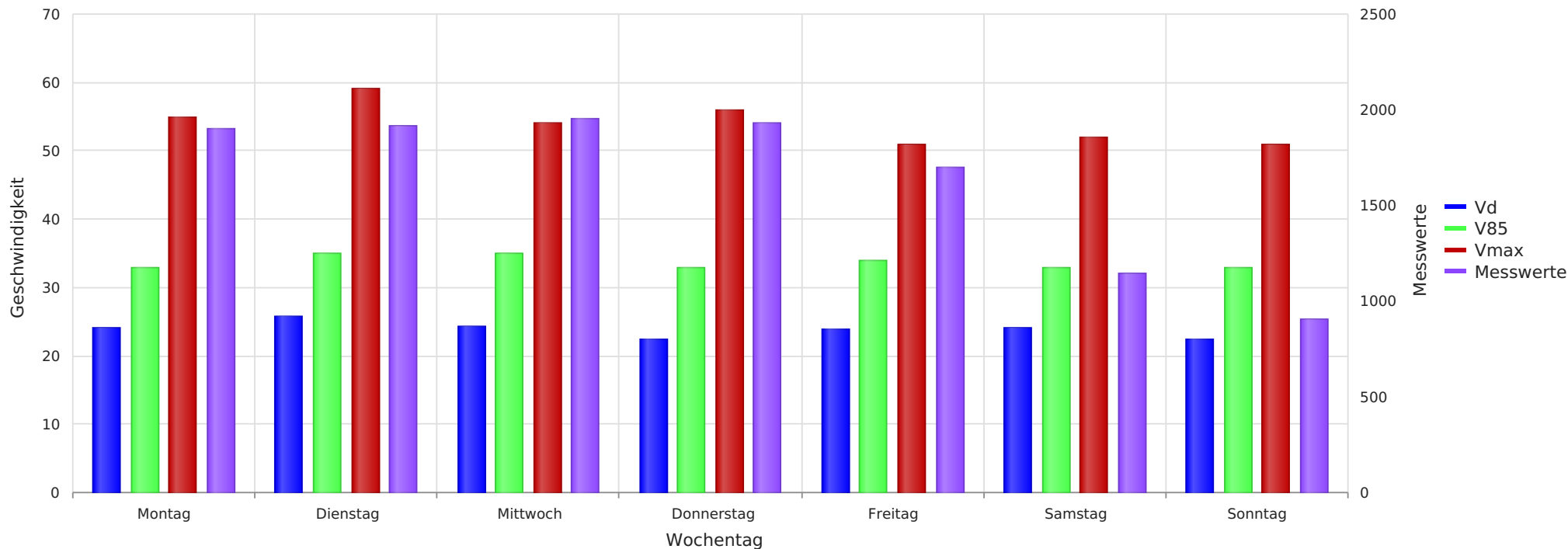
Am Mönckeberg, beide Fahrrichtungen, 30 km/h Beschränkung Vd, V85, Vmax, Anzahl der Messwerte vs. Wochentag
