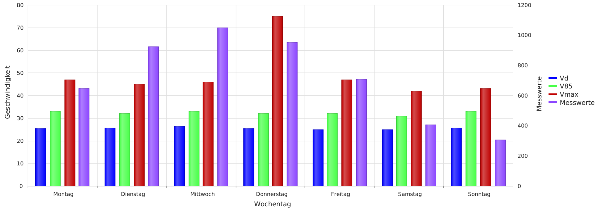
Am Wehrgraben (Velber) Richtung Gartenstr., 30 km/h Vd, V85, Vmax, Anzahl der Messwerte vs. Wochentag
