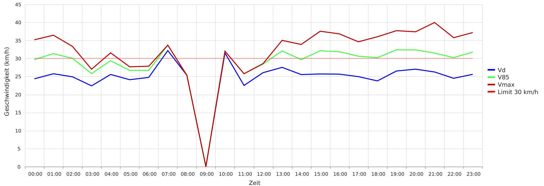
Am Wehrgraben (Velber) Richtung Gartenstr., 30 km/h Vd, V85, Vmax vs. Uhrzeit
